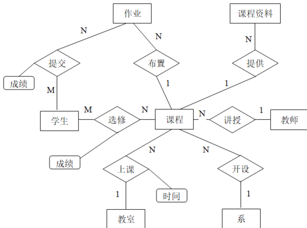
教学管理局部应用 E-R 图
