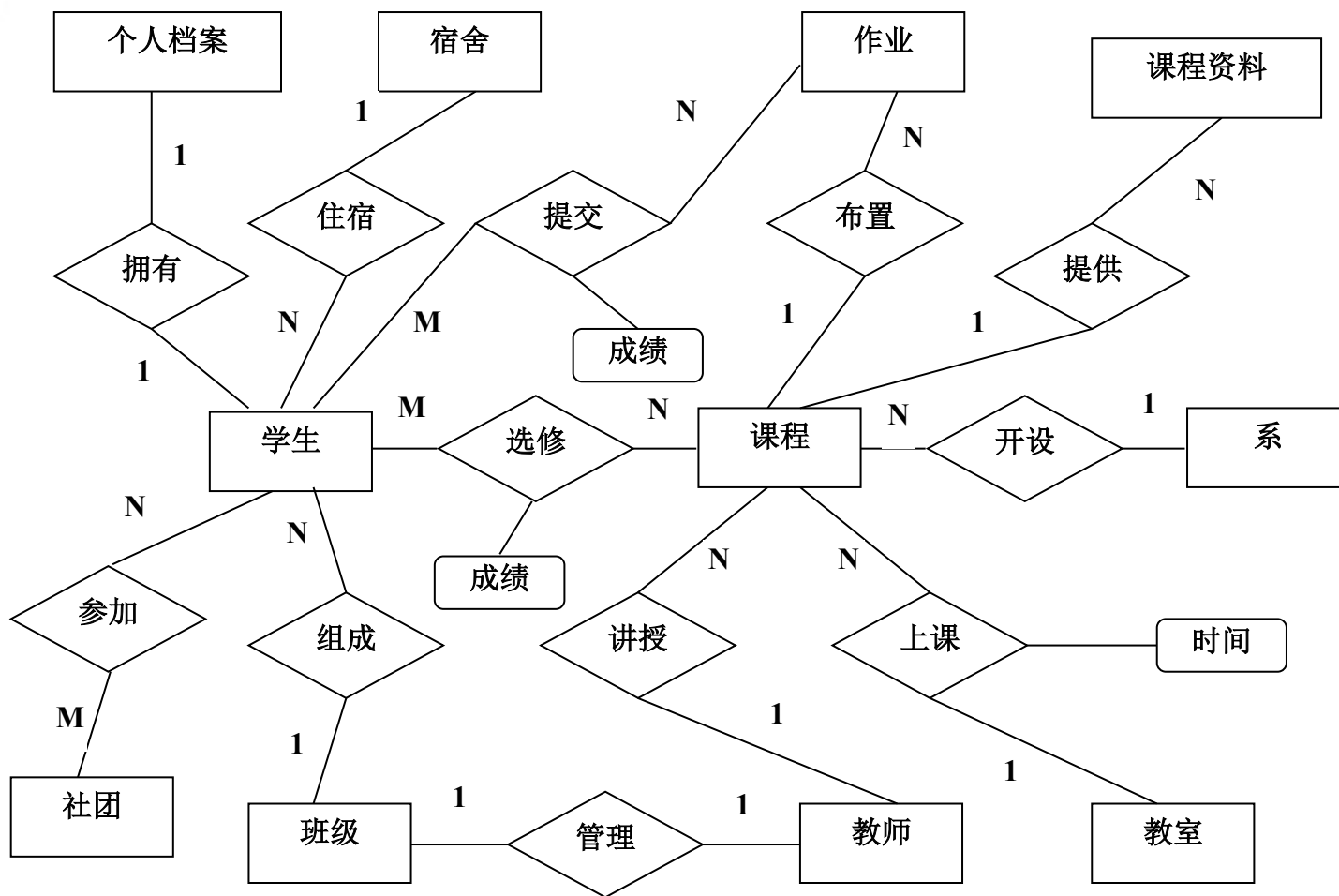
全局E-R图
